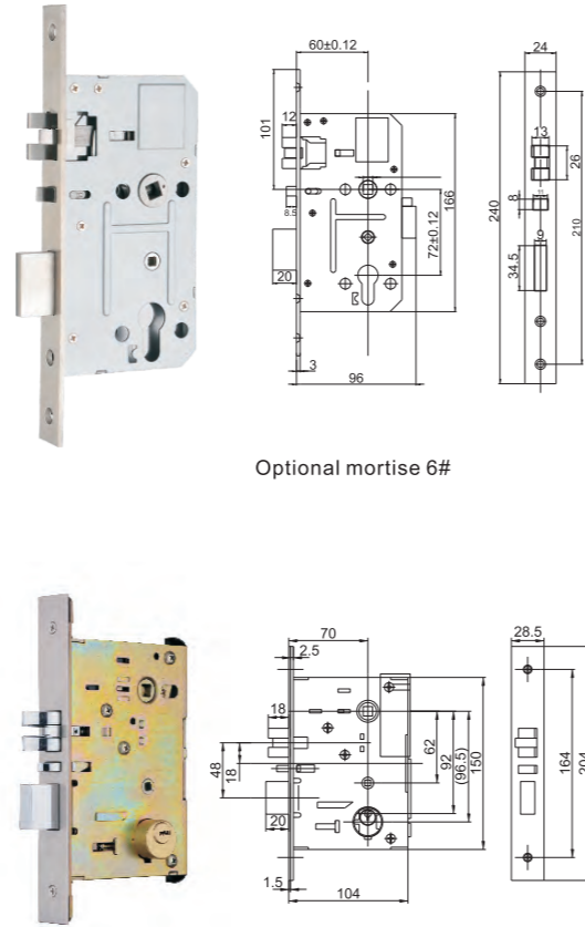
Standard mortise ANSI
