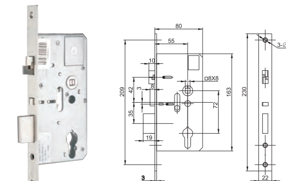
Optional mortise 3#
