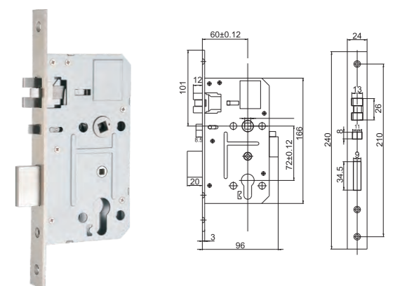
Optional mortise 6#
