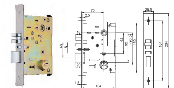
Standard mortise ANSI
